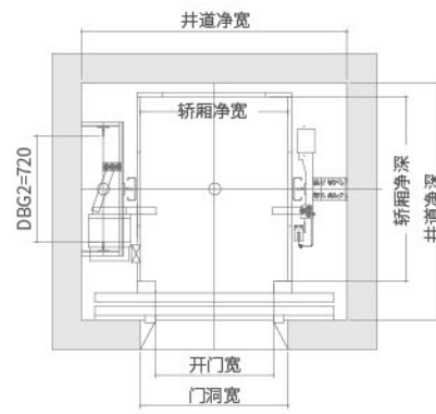
井道平面布置图 (中分门)
