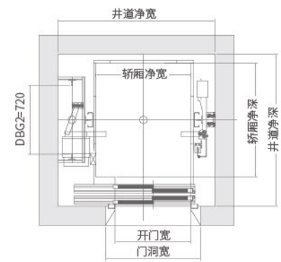
井道平面布置图 (旁开门)
