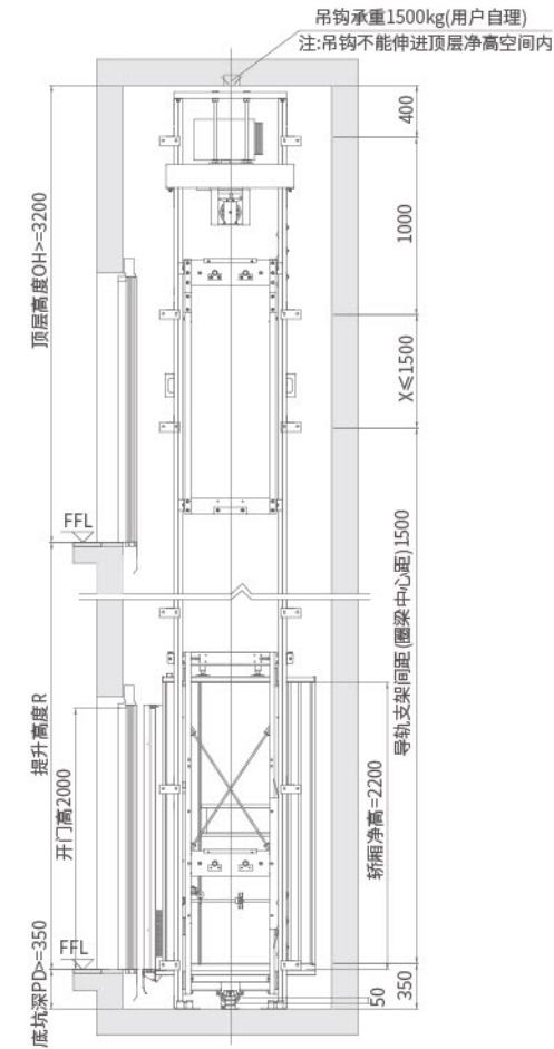
井道剖面图 JJ
