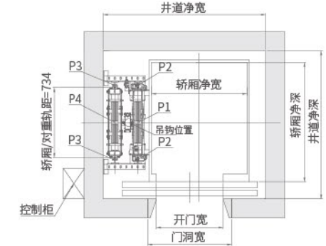
井道平面布置图 (中分门)
