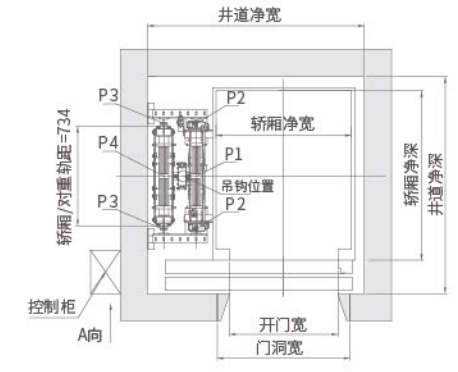
井道平面布置图 (旁开门)
